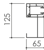
Guida plus con compensatore 125
