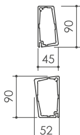
Profilo bracci
