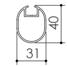
Profilo K40
