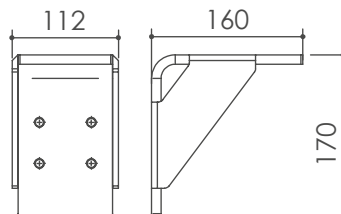
Staffa a L per attacco a soffitto 144 €/cp
