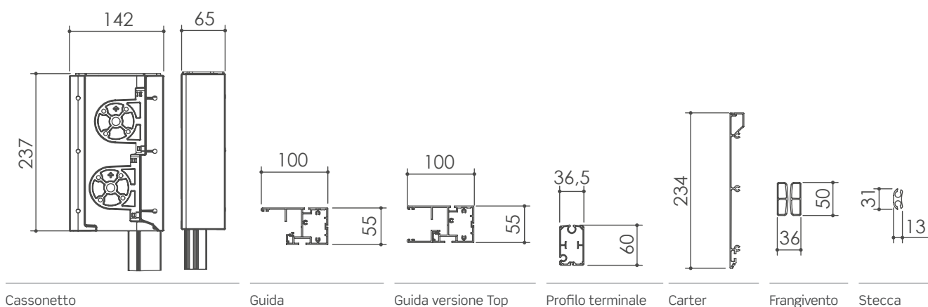
Cassonetto
