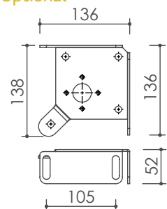
Staffa inox
