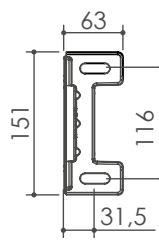
Staffa attacco a parete/soffitto
