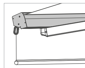
Volant a rullo (fino a max 6 m): Terminale con cassonetto e volant a rullo supplementare (h 150 cm) azionabile tramite argano, ideale per una migliore protezione dal sole.
