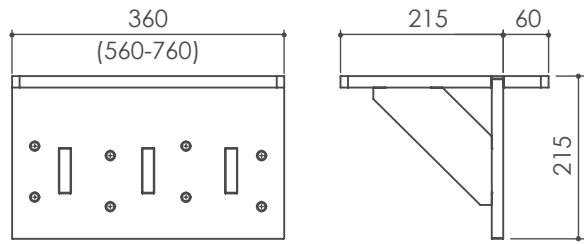
Controstaffa a soffitto
