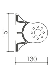
Staffa attacco a parete/soffitto
