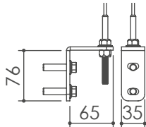
Staffa in acciaio per fissaggio cavi P 65mm
