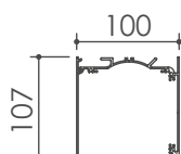
Cassonetto 100
