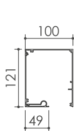
Cassonetto 100
