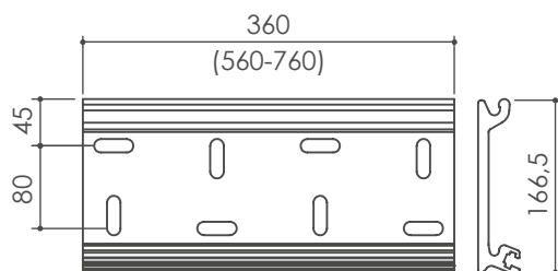
Staffa di premontaggio
