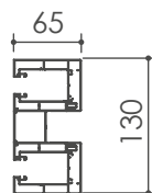
Guida plus (Std per versione con Cristal)
