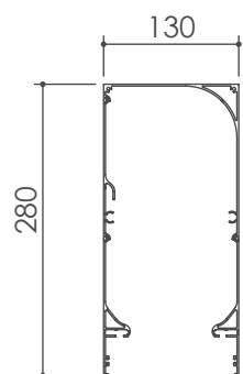
Cassonetto 100
