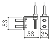
Staffa in acciaio per fissaggio cavi P 58mm
