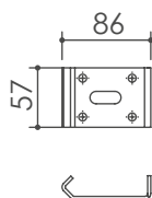
Staffe per montaggio a soffitto
