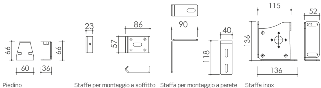
Piedino
