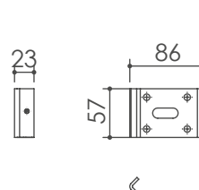
Staffe per montaggio a soffitto
