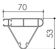
Profilo K70R
