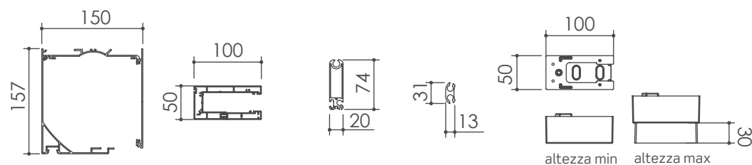
Cassonetto
