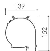
Cassonetto Round
