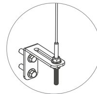
Dettaglio staffe in acciaio
