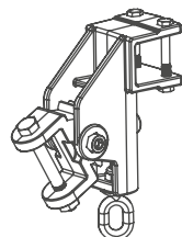
Attacco braccio a cremagliera (fino a max 6 m): Per una facile regolazione dell'inclinazione sia da parte del posatore che dell'utilizzatore finale.
