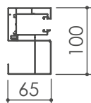
Guida plus con compensatore 100
