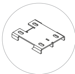
Dettaglio staffa
