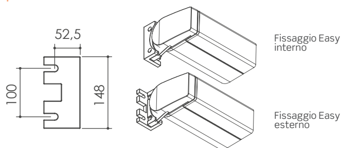
Staffa per attacco soffitto/parete (VERSIONE EASY)
