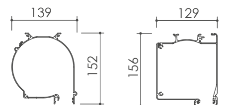
Cassonetto Round
