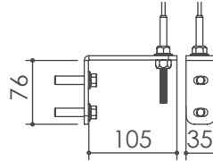
Staffa in acciaio per fissaggio cavi P 105mm
