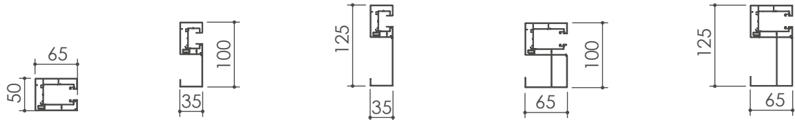
Guida plus (Std per versione ad argano e con Cristal) Guida con compensatore 100 Guida con compensatore 125 Guida plus con compensatore 100 Guida plus con compensatore 125
