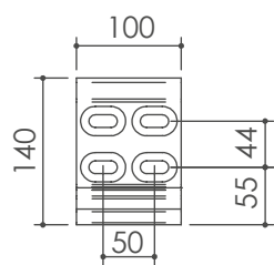
Supporto parete/soffitto
